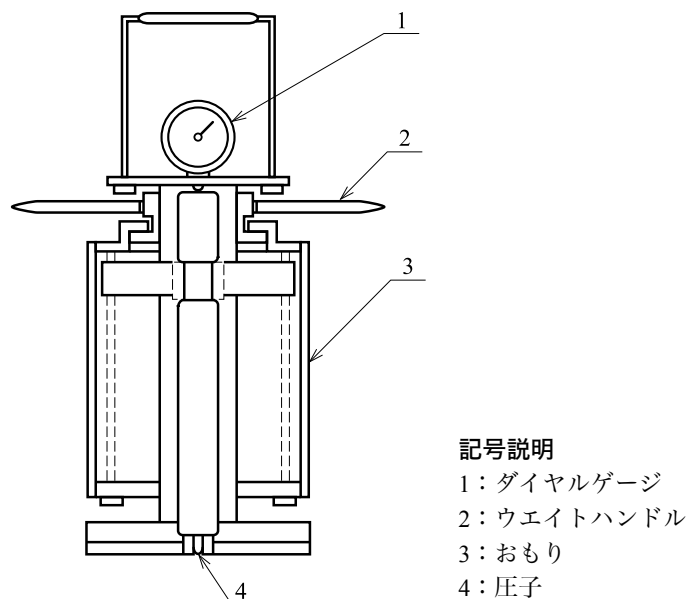
図 7—へこみ試験機の場合
