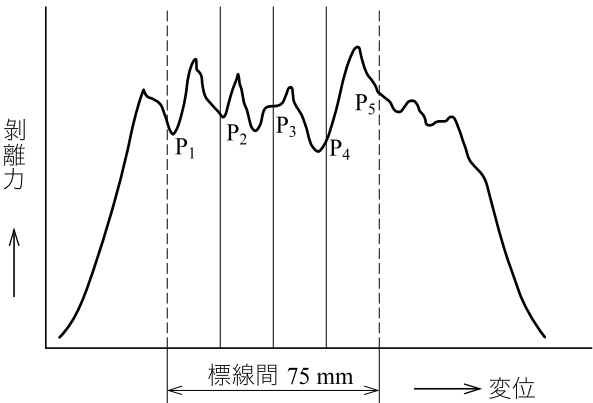
図 23－剥離力曲線の例
