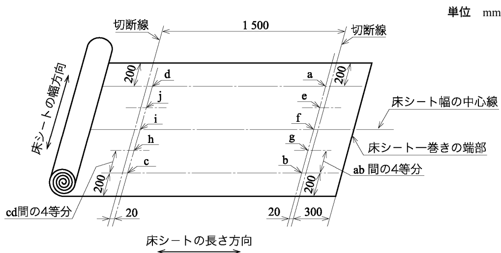
図 6 床シートの厚さの測定箇所
